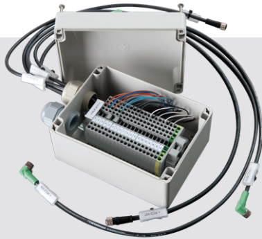
Bestückte Standardgehäuse Assembled standard enclosures
